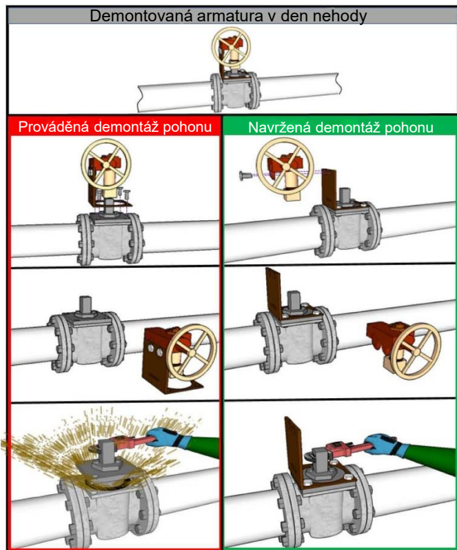
Obrázek 1: Znárodnění správného a chybného způsobu demontáže ručního kola armatury popisované nehody (Zdroj: Figure 3 CSB report 2016-02-I-LA)
