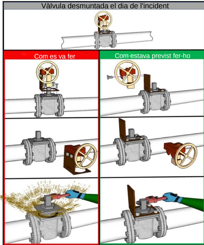
Figura 1: Diagrama que mostra les formes correcta i incorrecta de desmuntar el volant descrites a l'incident (Ref. Figura 3 de l'informe 2016-02-I-LA del CSB)
