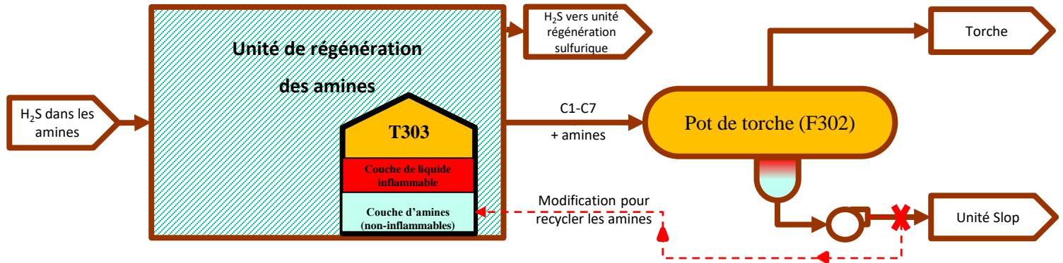
Figure 1. Flux originaux. Des aminés partent vers l'unité Slop
