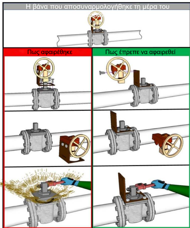
Εικόνα 1: Διάγραμμα που απεικονίζει τον σωστό και τον λανθασμένο τρόπο αφαίρεσης του μηχανισμού χειρισμού που περιγράφεται στο συμβάν (Πηγή: Εικόνα 3 CSB report 2016-02-I-LA )
