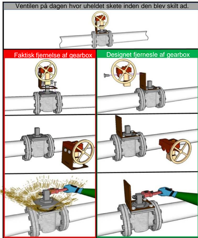
Figur 1: Diagrammet viser korrekt og forkert måde at fjerne håndhjulet på, som beskrevet i uheldsrapporten (Ref. Figur 3 CSB rapport nr. 2016-02-I-LA)
